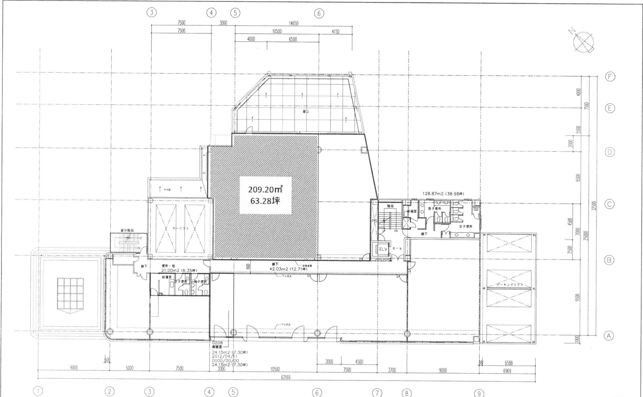
2階平面図
