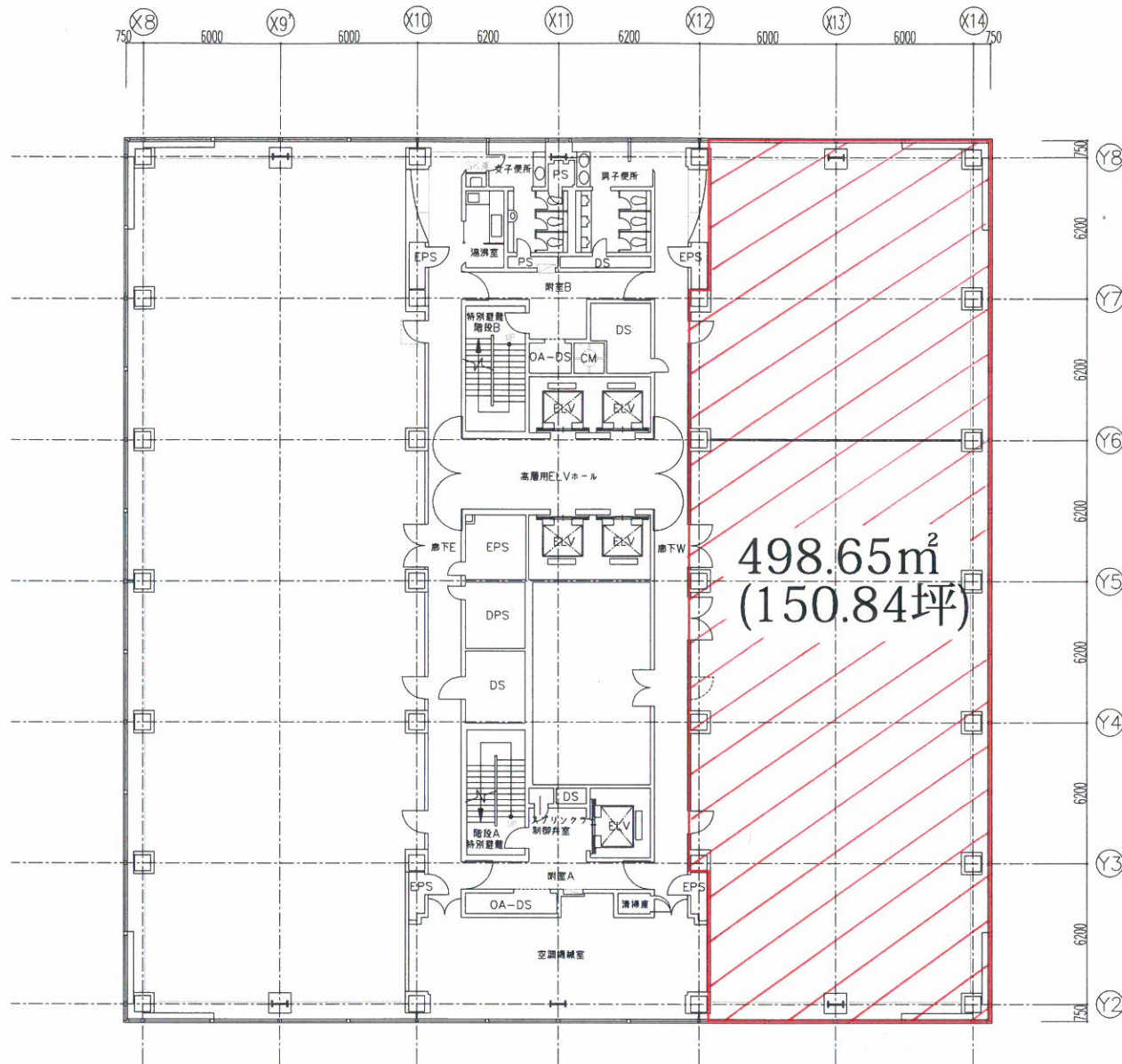
16階平面図
