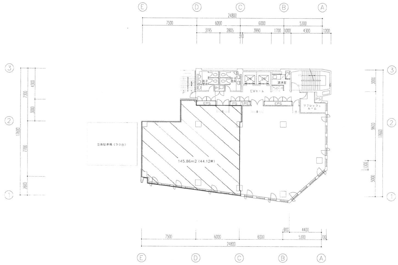
5階平面図
