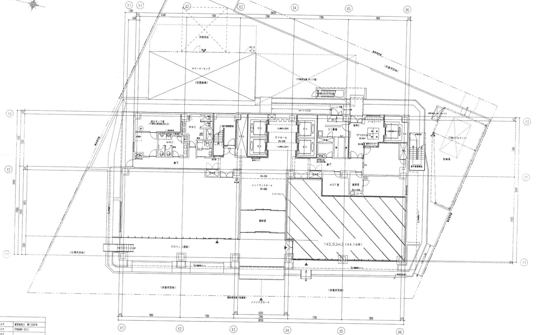
1階平面図
