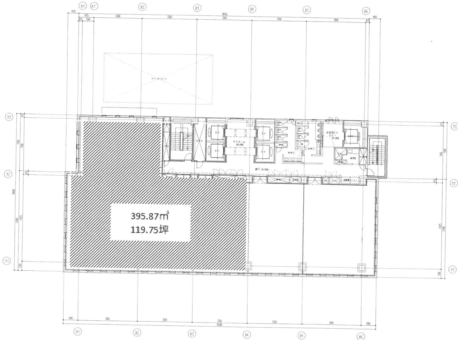
12階平面図
