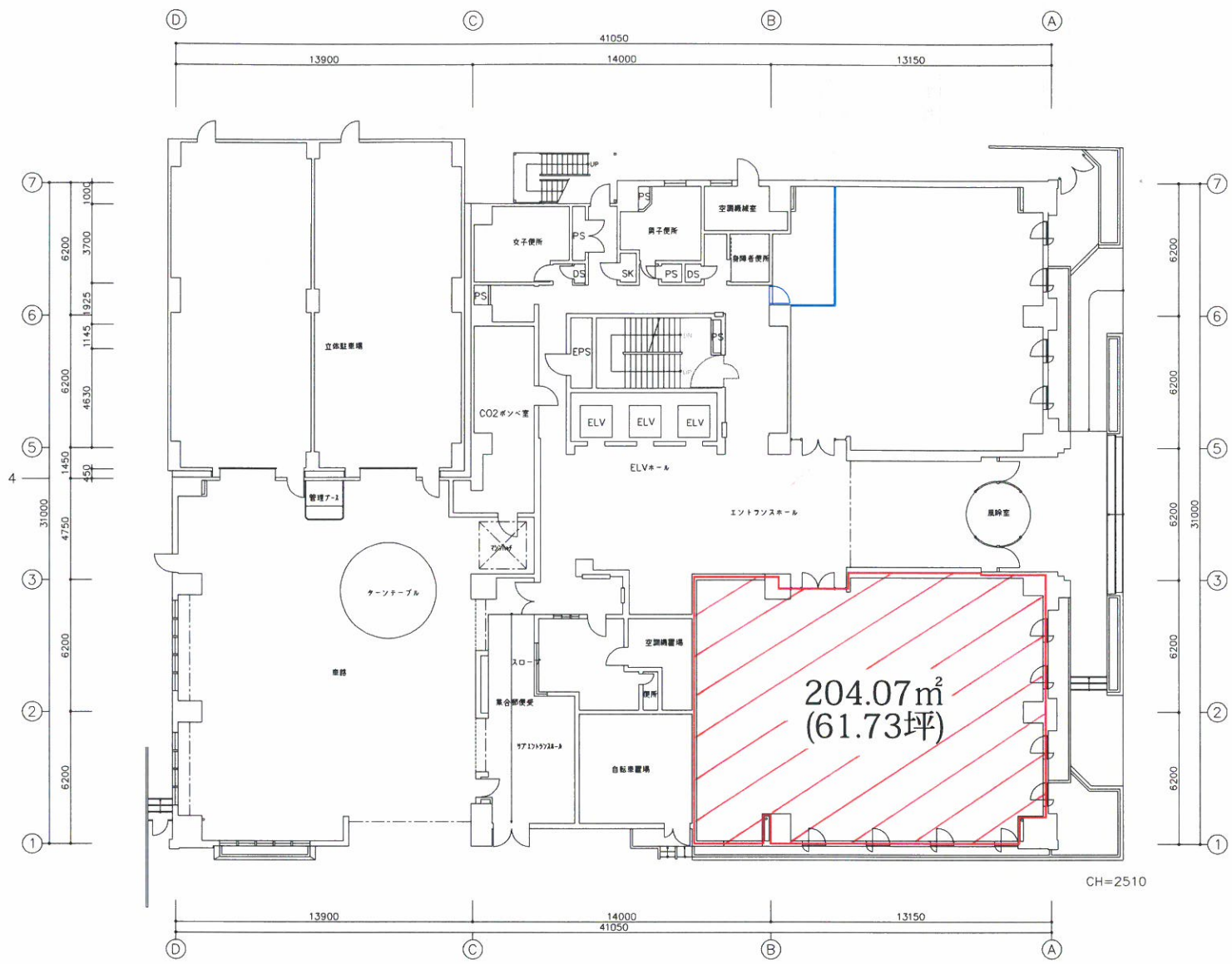
1階平面図
