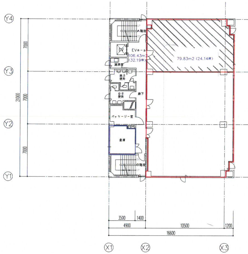
7階平面図
