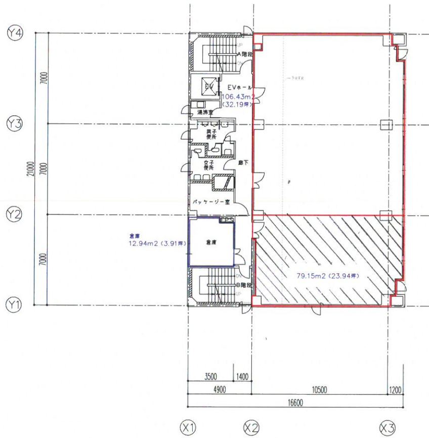
6階平面図
