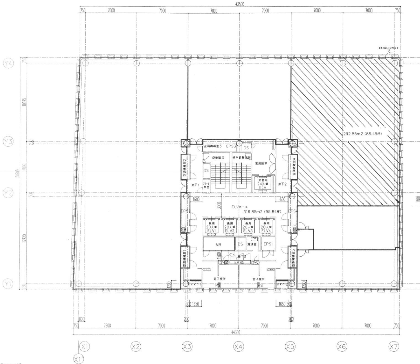
10階平面図
