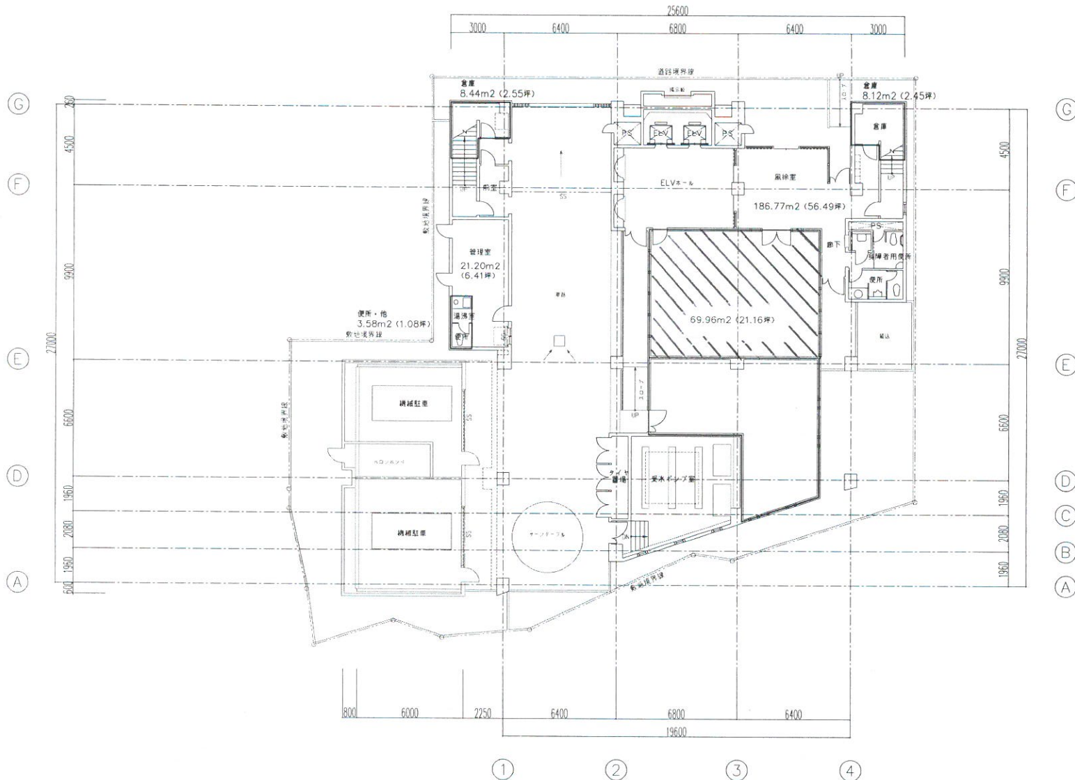
1階平面図
