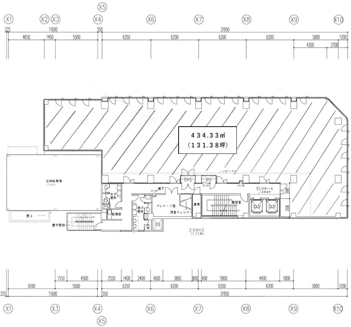
2階平面図
