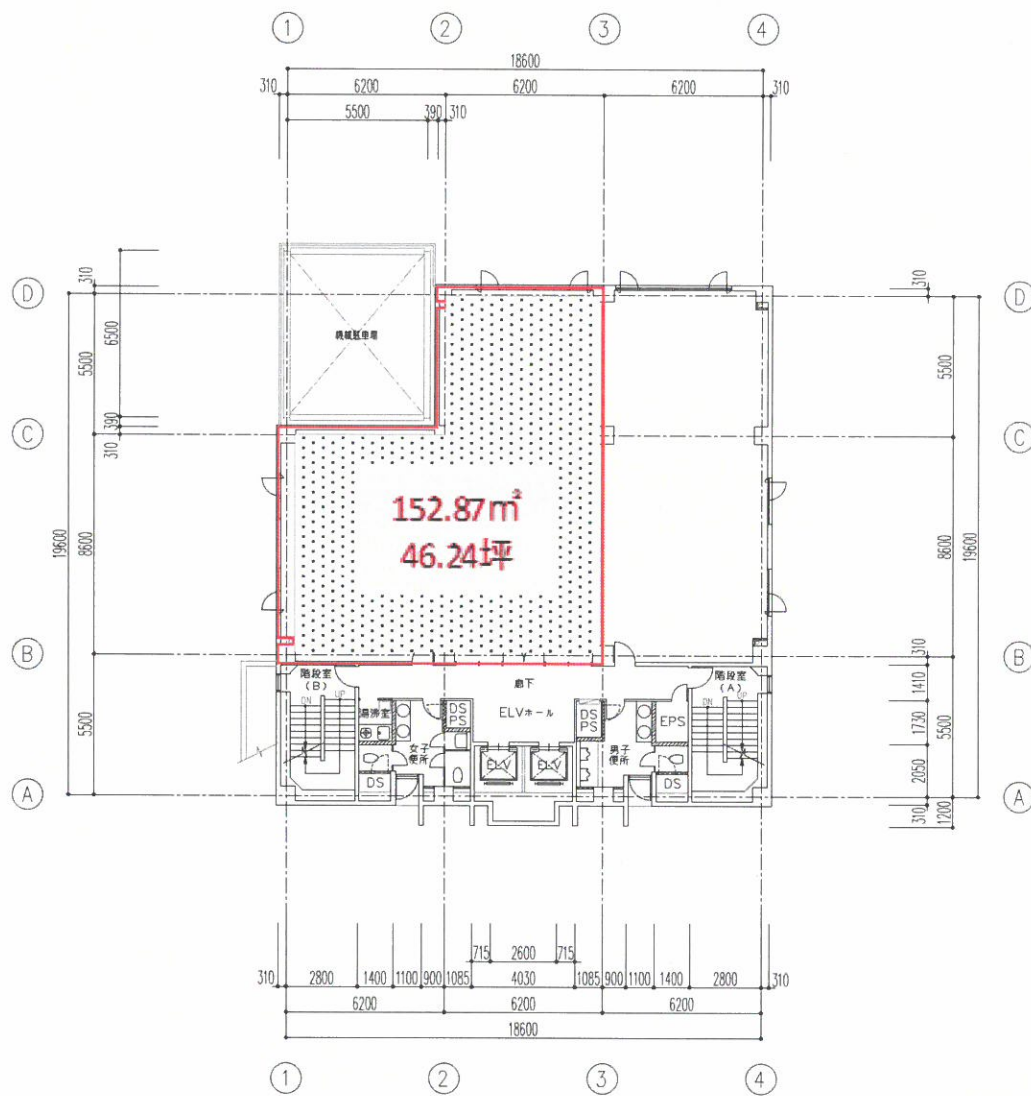
3階平面図
