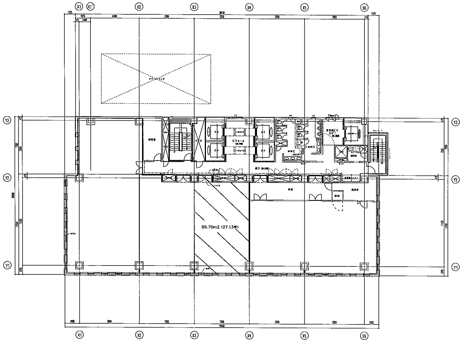
9階平面図
